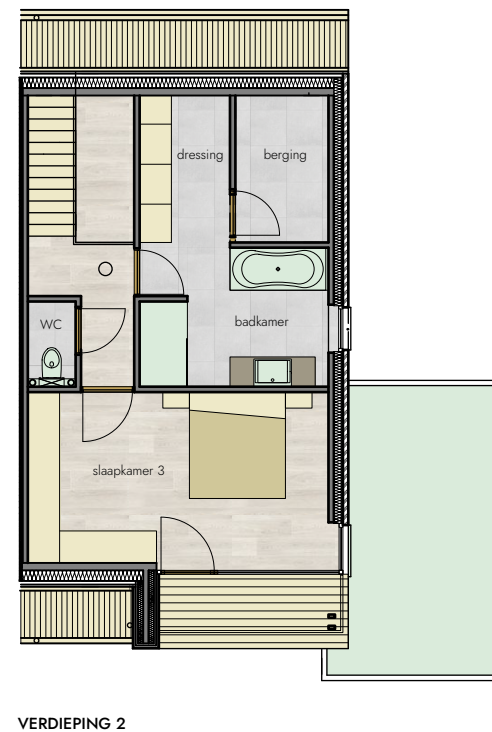
VERDIEPING 2
